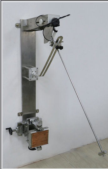
Equipo de prueba para IK04 a IK06
