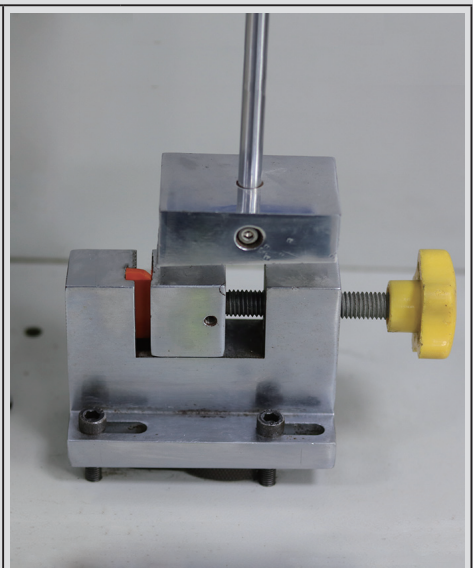
Espécimen después de la verificación Charpy
