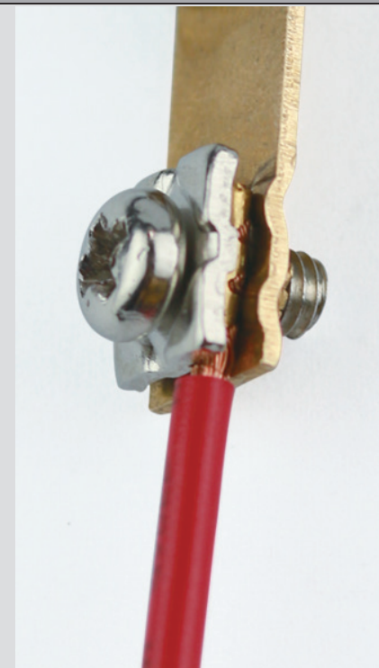
Detalle del terminal
